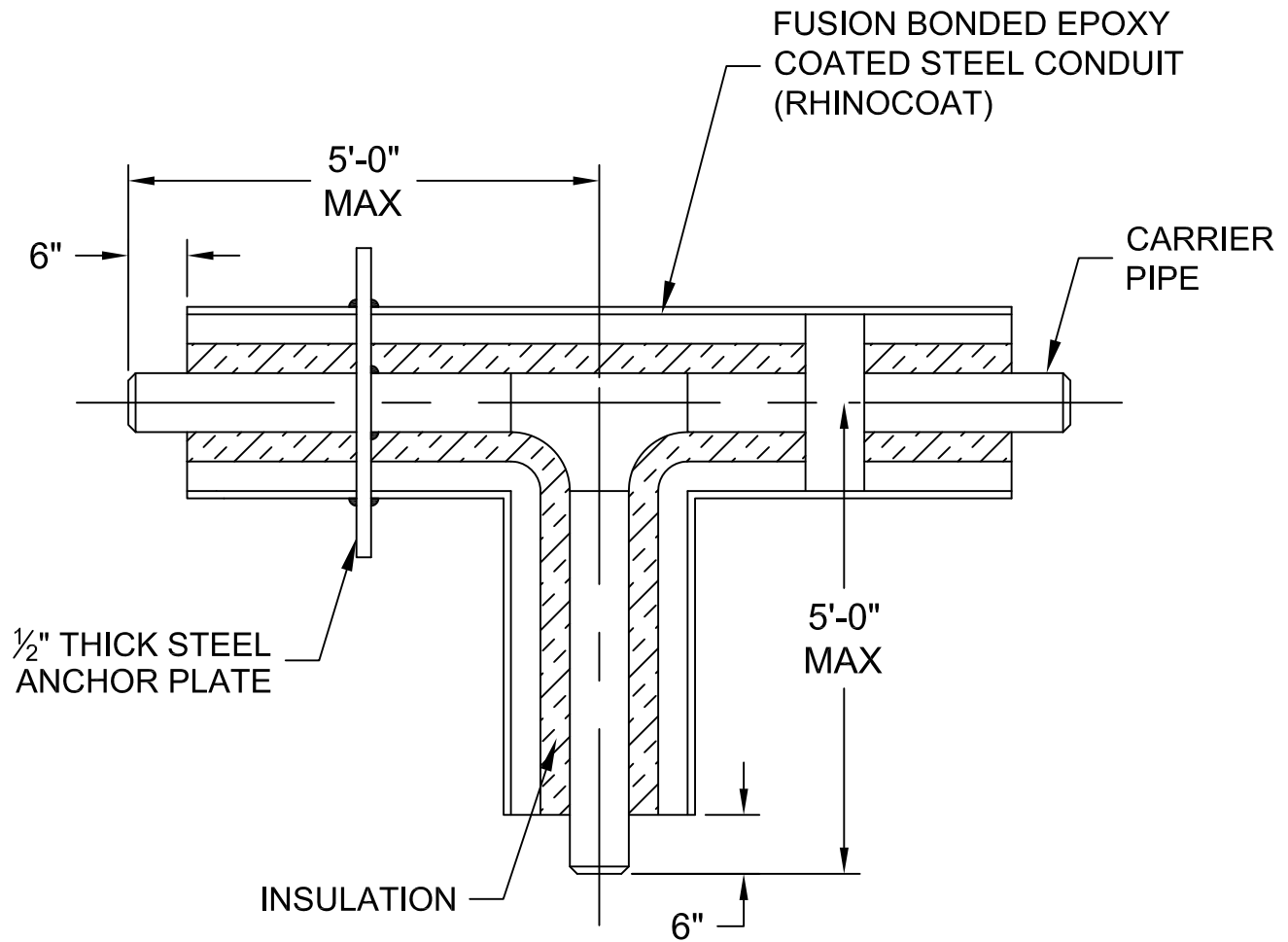
CONDUIT TEE W/ANCHOR DETAIL
