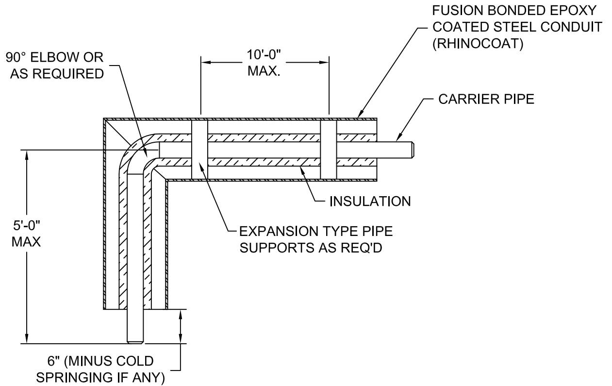
CONDUIT MITERED ELBOW DETAIL
